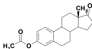
Estrone acetate
